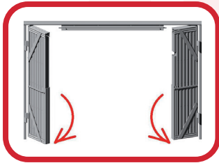
Modelo 1 Dos hojas exteriores
